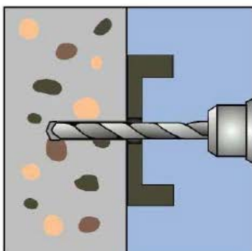
Poraa reikä
