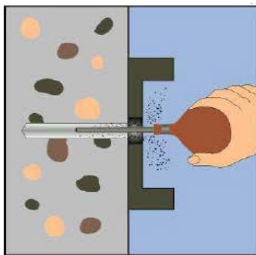
Puhdista reikä
