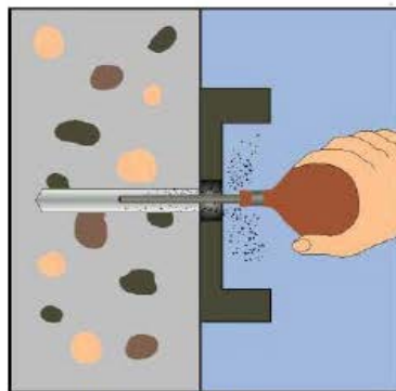
Puhdista reikä
