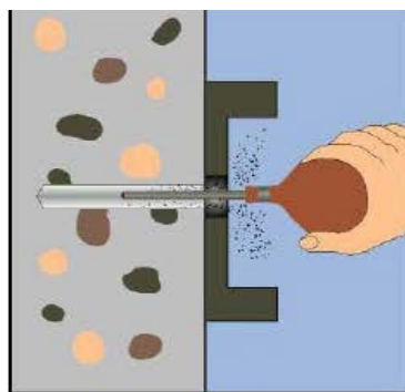
Puhdista reikä
