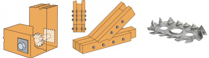
Embrèvement d'une ferme.
